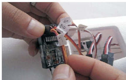
17. Connectez l'ESC et les servos au récepteur. Voir les instructions pour plus d'rayon pour les canaux appropriés et la polarité des prises de servo.
