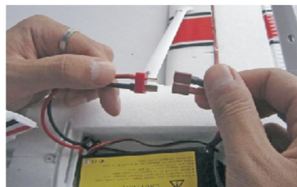
18. Placez la batterie dans son compartiment et connectez l'ESC.
