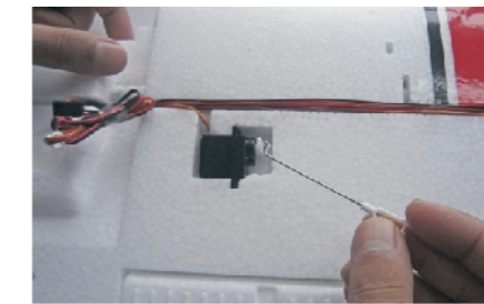
2. Connectez le poussoir au bras servo du aileron (premier trou).
